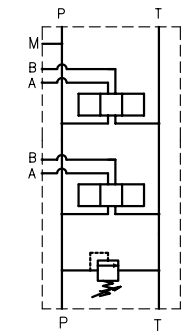
Schema idraulico in parallelo Schema hydraulique parallele
